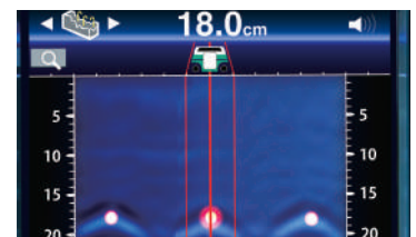
Έγχρωμη οθόνη LCD 4,1". Λειτουργία απλής και πολλαπλής ανίχνευσης αντικειμένων (εμφάνιση έως και 3 αποτελεσμάτων εντοπισμού στην οθόνη κάθε φορά)
